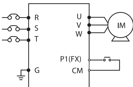
[Schemat połączeń]
